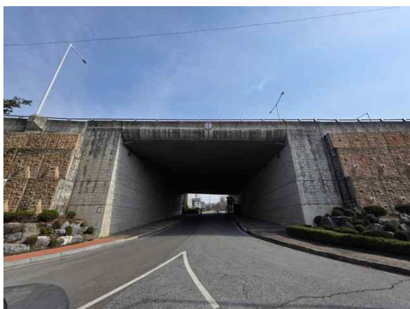
영룡1교 측면전경
